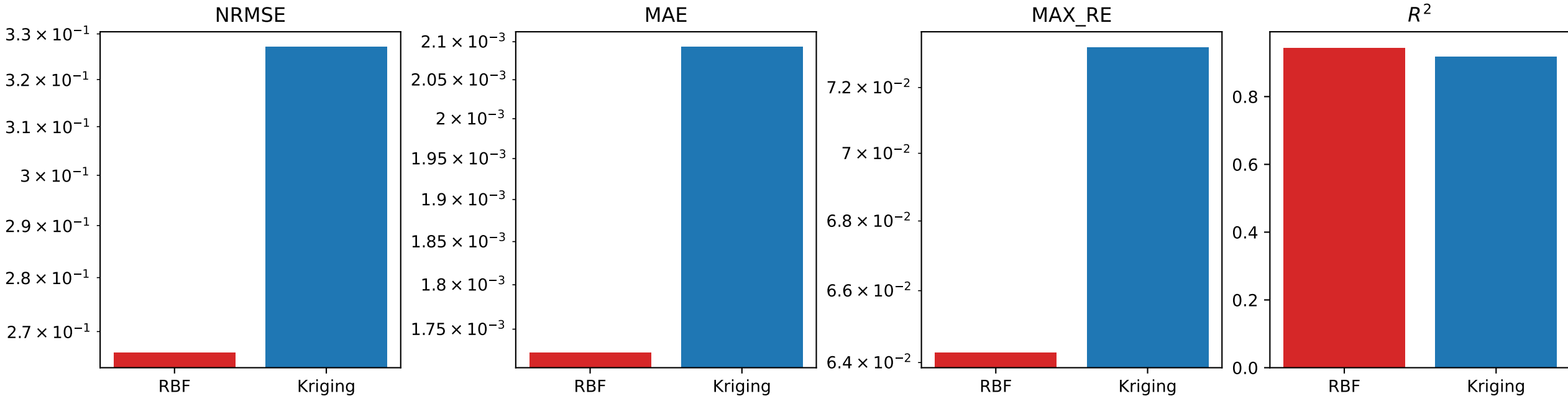
Якість RBF vs Kriging при n_s = 50 на Heat-AMIcon / q
